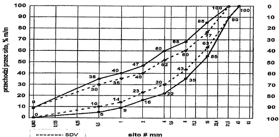
Rysunek 1. Uziarnienie mieszanek kruszyw przeznaczonych do warstw podbudowy 0/31.5.
