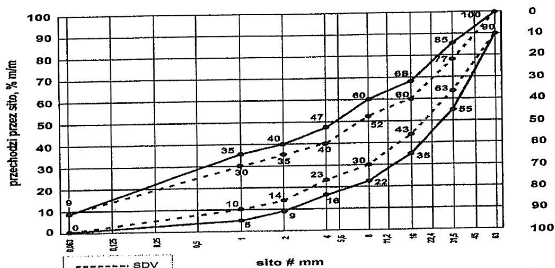
Rysunek 2. Uziarnienie mieszanek kruszyw przeznaczonych do warstw podbudowy 0/63.
